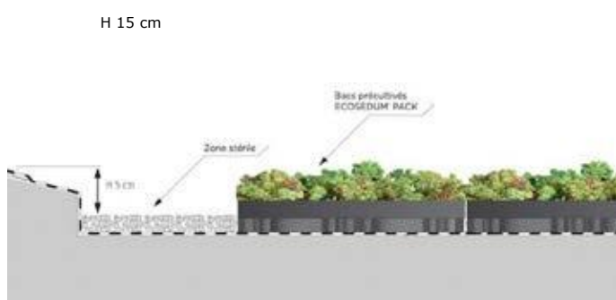
Système ECOSSEDUM PACK et zone stérile en gravillons
